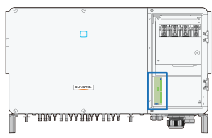
RS485-Schnittstelle (Klemmenblock)
