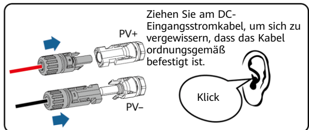
DC-Eingangsklemmen
